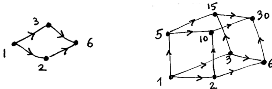
Figure 7. Diagramme de Hasse des diviseurs de 6 et des diviseurs de 30 pour la relation "divise" \mid . On remarque qu'on retrouve le diagramme de gauche au sein de la figure de droite puisque D(6) \subset D(30) .
